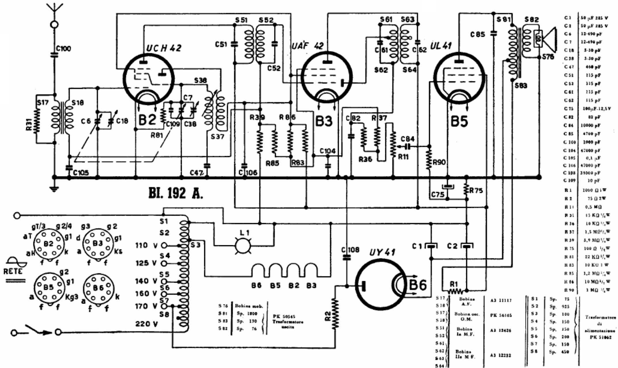
PHILIPS RADIO - Mod. BI 192 A. Questo schema vale per gli apparecchi sino al n. 127 601. OM da 550 a 1630 kc. Media frequenza 468 kc/s. Corrente totale anodica 66 mA cc. Consumo totale 28 watt.
